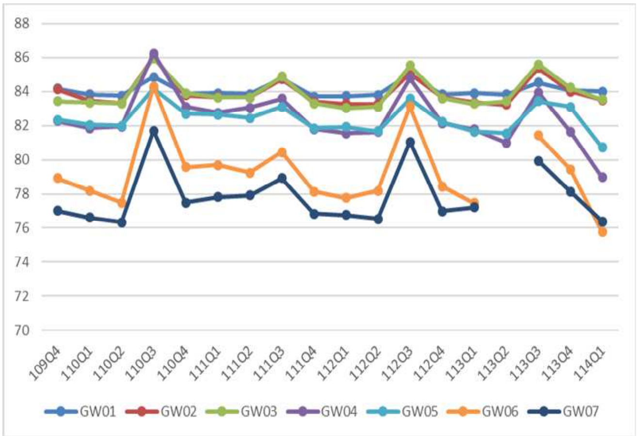
圖 4-4 109Q4~114Q1 地下水監測井水位監測變化圖
